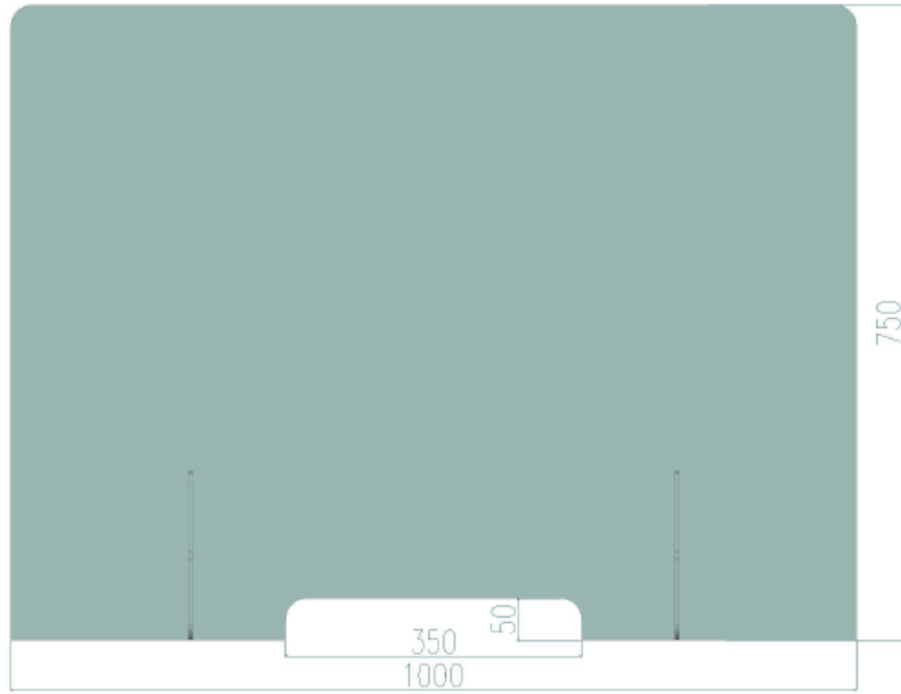
VISTA FRONTALE
